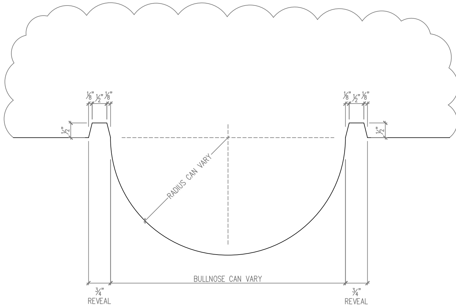
- BULLNOSE DETAIL SCALE: 6" = 1'-0"
